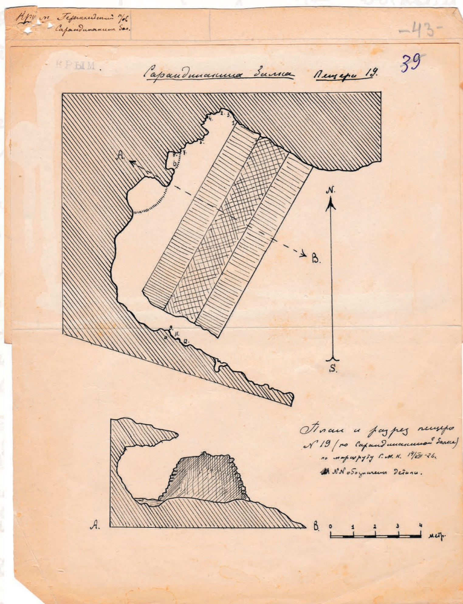
Материалы Севастопольского музея краеведения. План и разрез башни № 19 (Сарандинакина балка). Чертил Евгений Веймарн. 1926 г.
